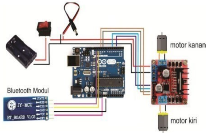
Gambar 1. Skema Rangkaian
