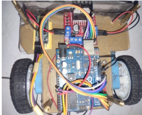
Gambar 3. Proses Rancangan Alat
