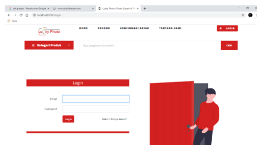
Gambar 7. Halaman Login
