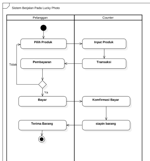
Gambar 2. Sistem berjalan
