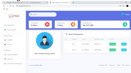
Gambar 8. Halaman utama
